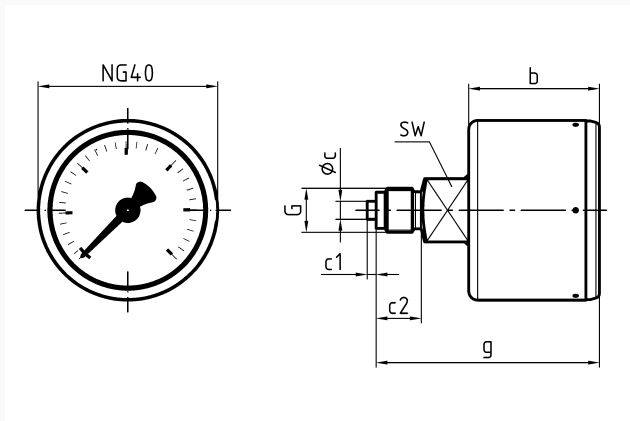
Maße (mm)
