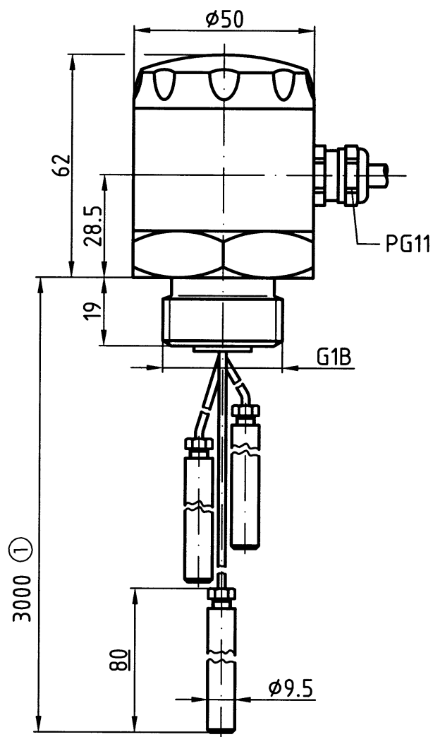
Seilsonde LSE 23
