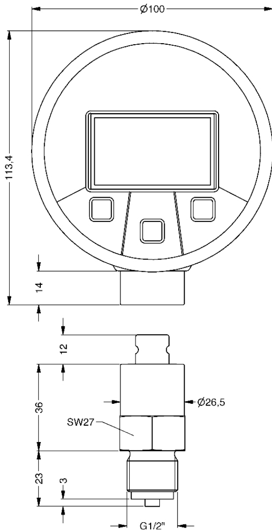
Digitalmanometer DIM 30
