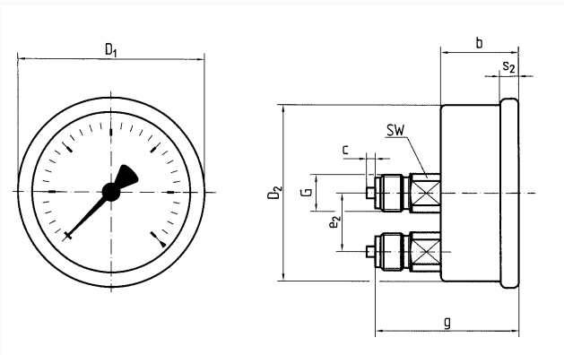
Maße (mm)
