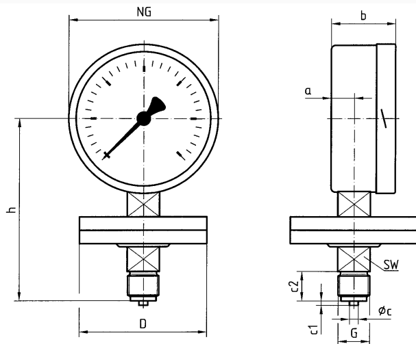
Maße (mm)
