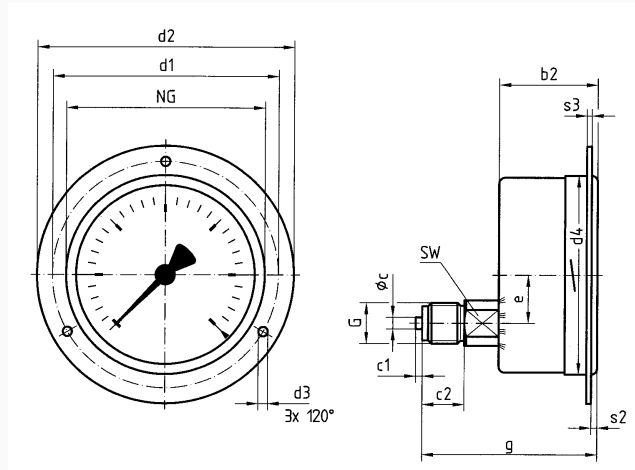
Anschluss axial exzentrisch, 3-Lochfrontflansch
