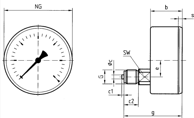
Maße (mm)
