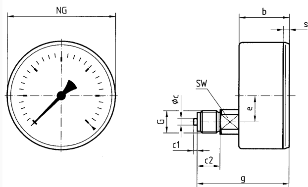
Maße (mm)
