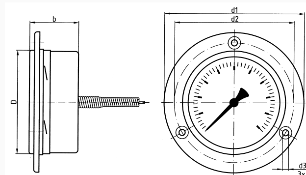
Ausführung mit Fernleitung und 3-Lochfrontflansch
