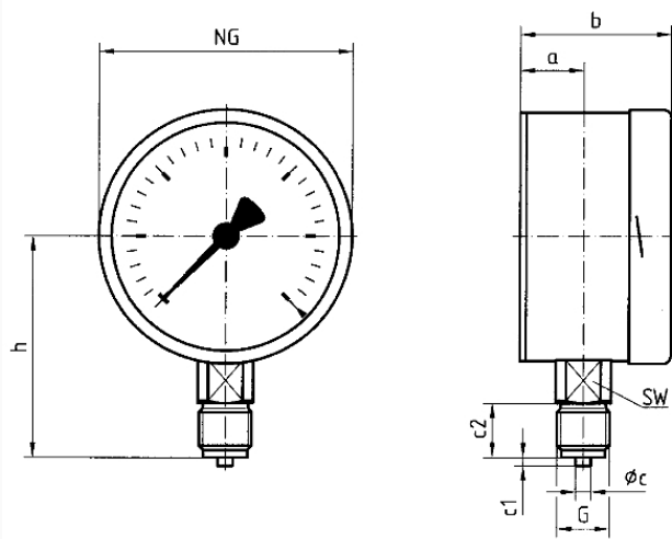
NG 100/160 – Anschluss radial
