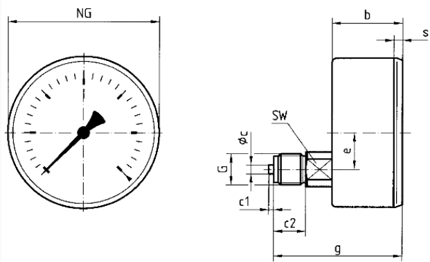
Masse (mm)
