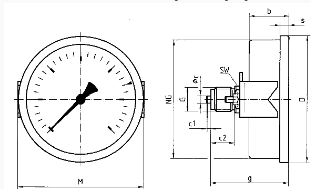
NG 100 – Anschluss axial, mit Bügelbefestigung
