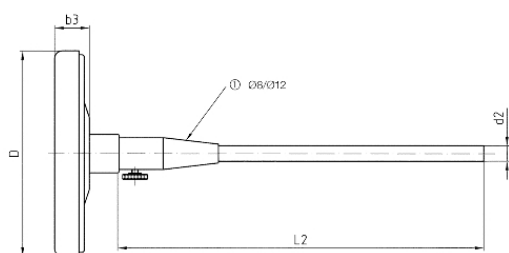
Anschluss axial
