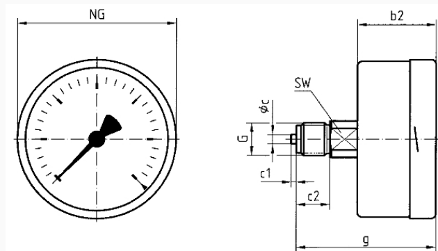
Anschluss axial
