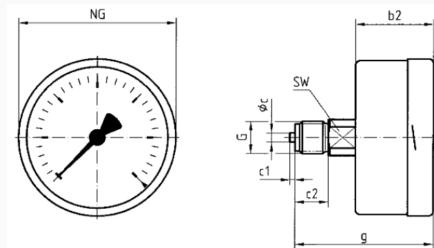
Masse (mm)
