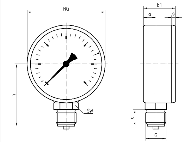
Masse (mm)
