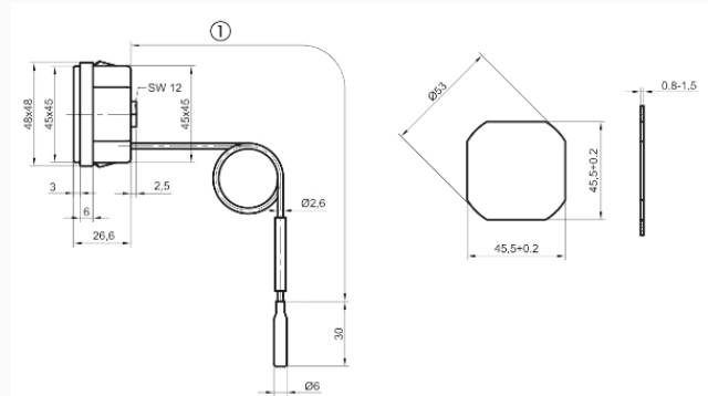
Typ THK 45
