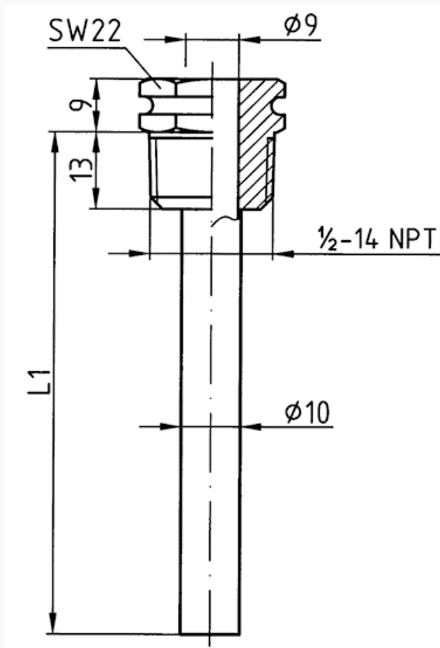
Tauchhülse ½" 9 x 10 mm
