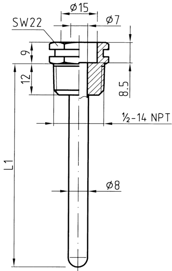
Tauchhülse 1/2" 7 x 8 mm
