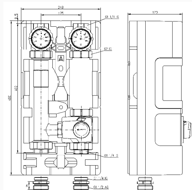
PrimoTherm® K 180-2 DN 32 KSV Vario
