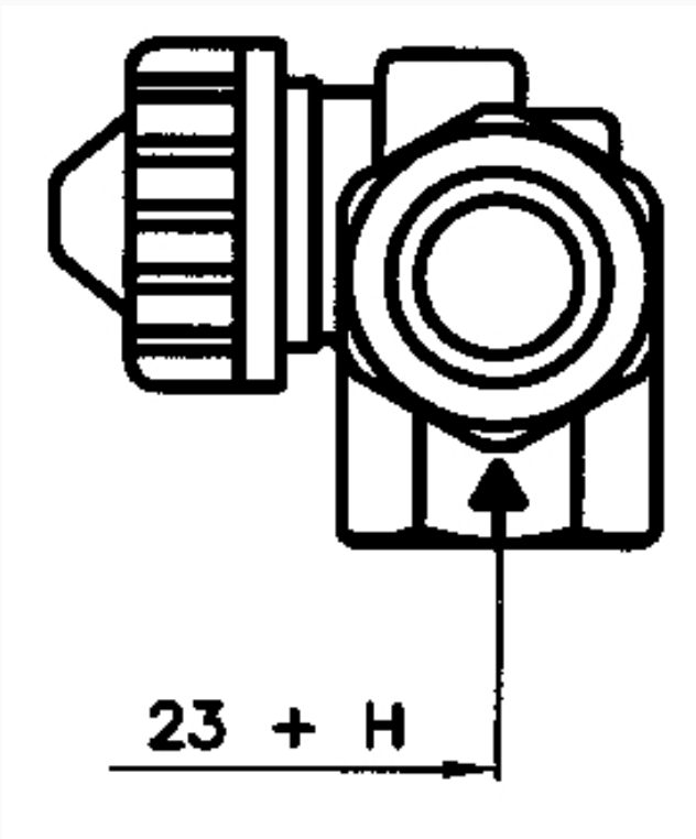
Masse (mm)
