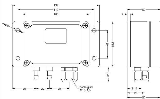
Differenzdruckmessumformer DMU 20 D
