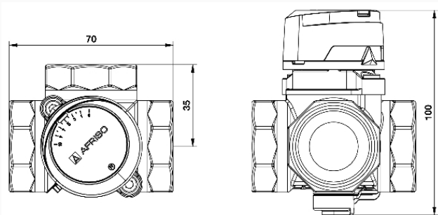
3-Wege-Mischventil DN 20
